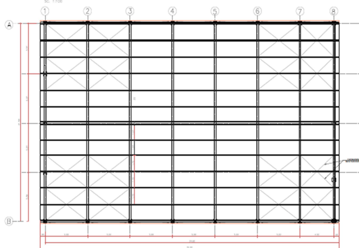
PLANTA DA ESTRUTURA DA COBERTURA
