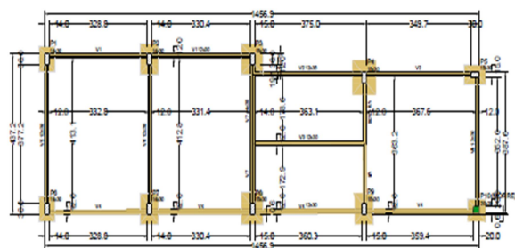
FORMA DO PAVIMENTO FUNDAÇÃO
