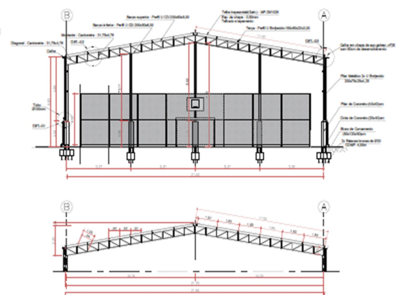
SEÇÃO DA TESOURA
