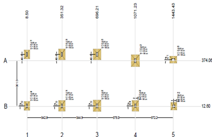
PLANTA DE LOCAÇÃO
