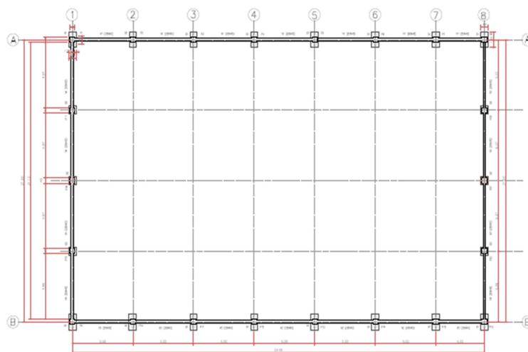
PLANTA DE LOCAÇÃO DA FUNDAÇÃO
